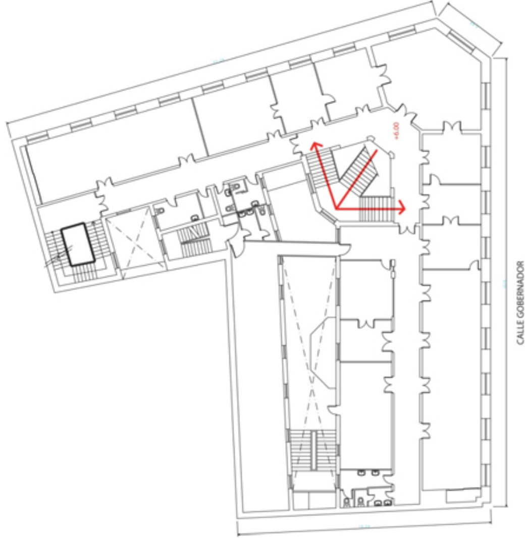
PRIMER PISO_1:200
